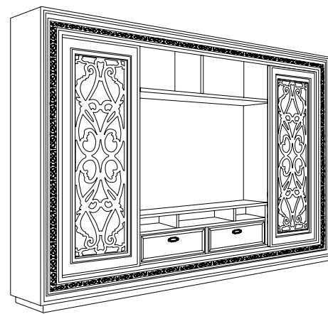
articolo F4000 parete soggiorno porta TV con ante traforate scorrevoli e cassetti con guida amortizzata. sitting room furniture TV stand with perforated sliding doors and drawers with soft closing. cm. l. 318 p. 47 h. 230 vano TV. TV comp. cm. l. 140 h. 108
