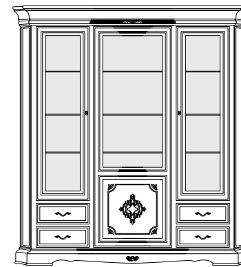
articolo E605 argenteria intarsiata, 3 porte, 4 cassetti con ripiani in cristallo. silver cabinet with inlay, 3 door, 4 drawers and crystal shelves cm. l. 203 p. 49 h. 220 smontabile. dismantles.
