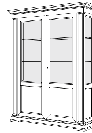
articolo E250 vetrina 2 porte con pannello liscio. showcase 2 doors with smooth panel. cm. l. 170 p. 45 h. 210 smontabile. dismantles.
