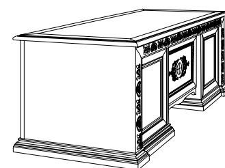
articolo E704 scrivania con cornicione intagliato sul lato anteriore e liscio sul lato posteriore e cassetto a ribaltina. writing-desk with carved front frame and smooth back frame with bureau drawer. cm. l. 185 p. 90 h. 80
