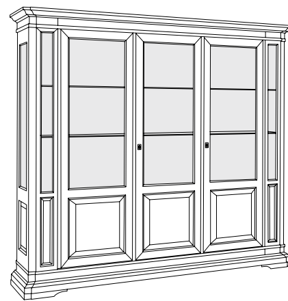
articolo E413 vetrina 3 ante con bugna. 3 beveled doors display cabinet. cm. l. 240 p. 48 h. 213 smontabile. dismantles.
