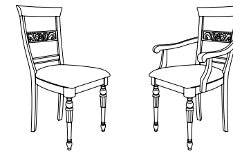
articolo E609 sedia con fondino tappezzato tipo C. chair with upholstered seat type C. cm. l. 48 p. 50 h. 96
