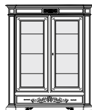
articolo E724 vetrina 2 porte con cassetto intarsiato. 2 door display cabinet with inlay. cm. l. 173 p. 50 h. 220 smontabile. dismantles.
