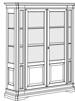
articolo E414 vetrina 2 ante con bugna. 2 beveled doors display cabinet. cm. l. 177 p. 48 h. 213 smontabile. dismantles.
