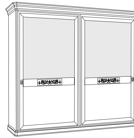
articolo E300/I armadio 2 ante scorrevoli con intarsio e vetri satinati. 2 sliding doors wardrobe with inlay and frosted glass. cm. l. 290 p. 67 h. 247
