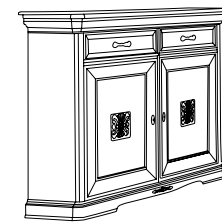
articolo E310 credenza 2 porte pannelli con intagli 2 cassetti. 2 doors sideboard with carvings panels 2 drawers. cm. l. 160 p. 55 h. 110
