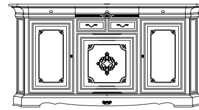
articolo E601 credenzone intarsiato, 3 porte e 4 cassetti. sideboard with inlay, 3 door and 4 drawers. cm. l. 220 p. 55 h. 115
