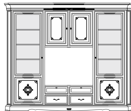
articolo E606 soggiorno intarsiato con ripiani legno. inlaid living room with wooden shelves. cm. l. 287 p. 49 h. 245 vano TV. TV compartment. cm. l. 103 p. 41 h. 84 smontabile. dismantles.
