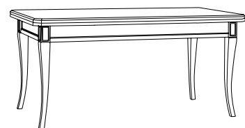
articolo E311 tavolo rettangolare allungabile 2 allunghe da cm 40. extendable rectangular table 2 extensions of 40 cm. cm. l. 170 p. 90 h. 80 aperto. open. 250 x 90 cm.
