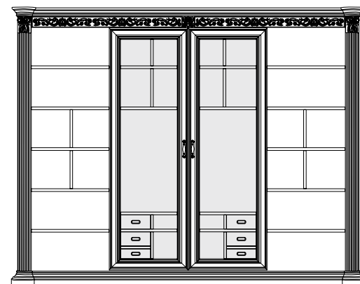
articolo E701 soggiorno a parete con ante scorrevoli, anta a vetro. sitting room with sliding doors with glass door. cm. l. 315 p. 47 h. 246 vano TV. TV compartment. cm. l. 135 p. 35 h. 91
