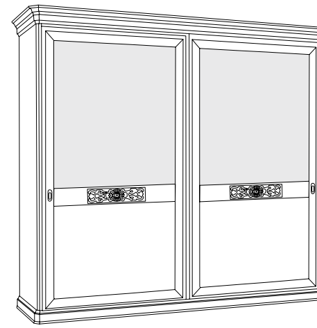
articolo E300 armadio 2 ante scorrevoli con intaglio e vetri satinati. 2 sliding doors wardrobe with carving and frosted glass. cm. l. 290 p. 67 h. 247
