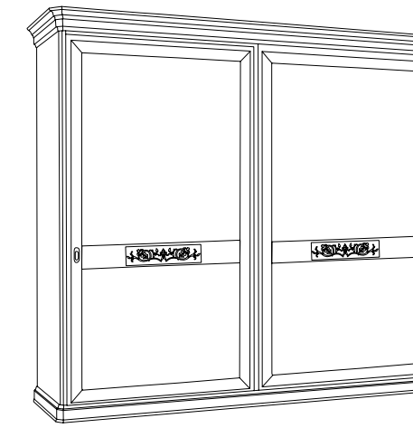
articolo E315/I armadio 2 ante scorrevoli con intarsio. 2 sliding doors wardrobe with inlay. cm. l. 290 p. 67 h. 247
