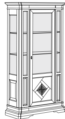
articolo E405 vetrina 1 anta con intarsio. 1 inlay door showcase. cm. l. 118 p. 48 h. 213 smontabile. dismantles.
