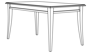
articolo E252 tavolo rettangolare allungabile 2 allunghe da cm 40. extendable rectangular table 2 extensions of 40 cm. cm. l. 160 p. 90 aperto. open. 240 x 90 cm.
