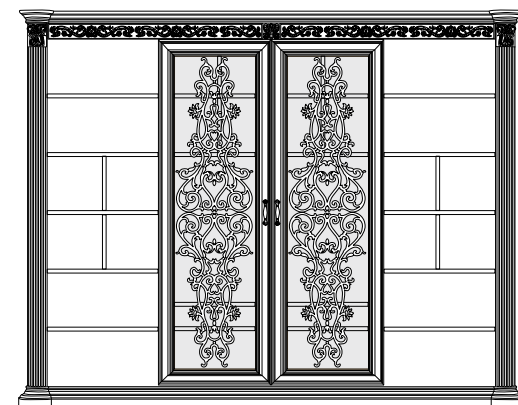
articolo E700 soggiorno a parete con ante scorrevoli, anta con traforo. sitting room with sliding doors with perforated door. cm. l. 315 p. 47 h. 246 vano TV. TV compartment. cm. l. 135 p. 35 h. 91
