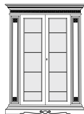
articolo PS15 argenteria 2 ante spalle con intaglio. 2 doors display cabinet carved shoulders. cm. l. 160 p. 48 h. 215,5 smontabile. dismantles.
