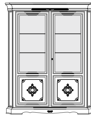
articolo E604 argenteria intarsiata, 2 porte con ripiani in cristallo. silver cabinet with inlay, 2 door and crystal shelves. cm. l. 176 p. 49 h. 220 smontabile. dismantles.
