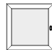
ART. EPS74 ANTA quadrata per vetro. cm. l. 59 sp. 2,8 h. 59
