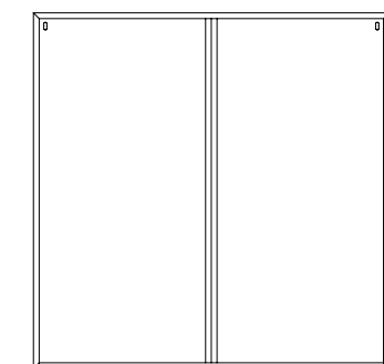
ART. CP/52 pensile cubo 2 vani. cm. l. 118 p. 36 h. 118
