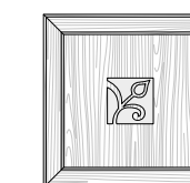
ART. SCM10 SX ANTA con intaglio per finitura noce. cm. l. 59 sp. 2,8 h. 59
