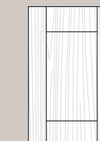
ART. CM41 anta a telaio legno verticale. cm. l. 36,6 h. 58,6 sp. 2,5
