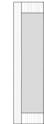
ART. EL/29 anta a telaio vetro verticale cm. l.36,6 h.117,6 sp.2,5
