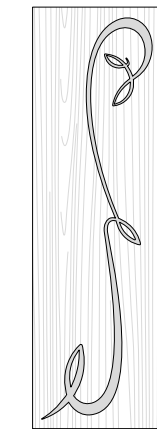
ART. EL/25SX anta con decoro verticale cm. l.36,6 h.117,6 sp.2,5
